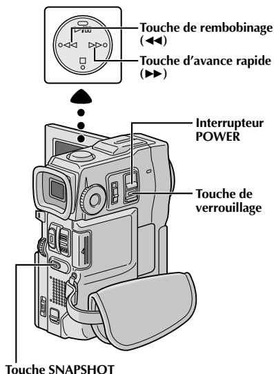
Affichage
